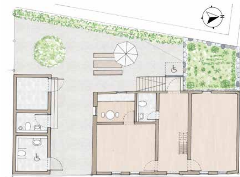
Nutzungskonzept Erdgeschoss, Variante 2, Maßstab 1:100. | Grafik: Architekturbüro Dipl.-Ing. Stephan Dreier, Architekten in der Baudenkmalpflege
