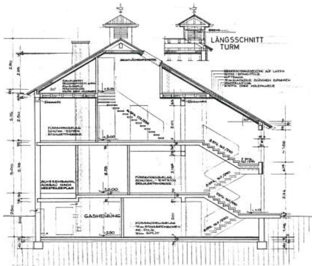
SCHNITT A-A
