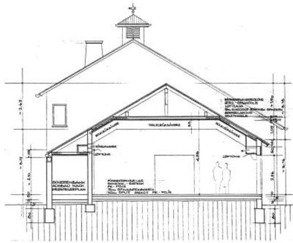
SCHNITT B-B
