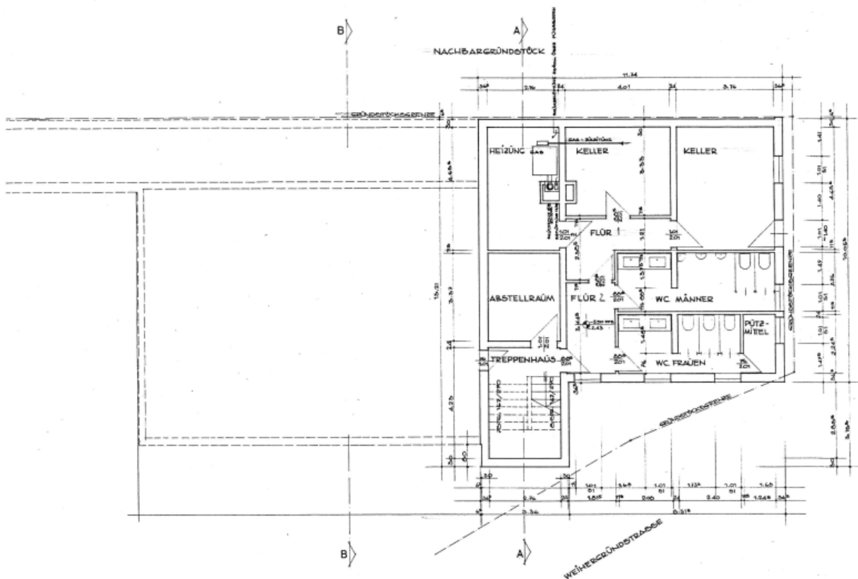
KELLERGESSCHOSS
